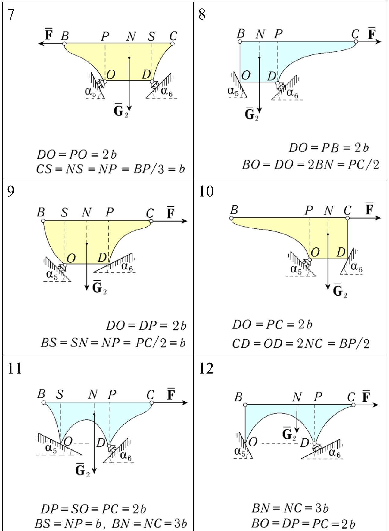
Рис. 24. Группа тел В для типового расчёта (структурные схемы 7–12)
