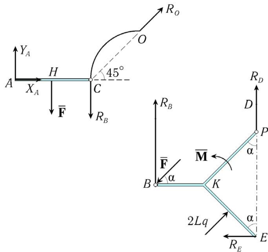
Рис. 18. Результат расчленения системы
