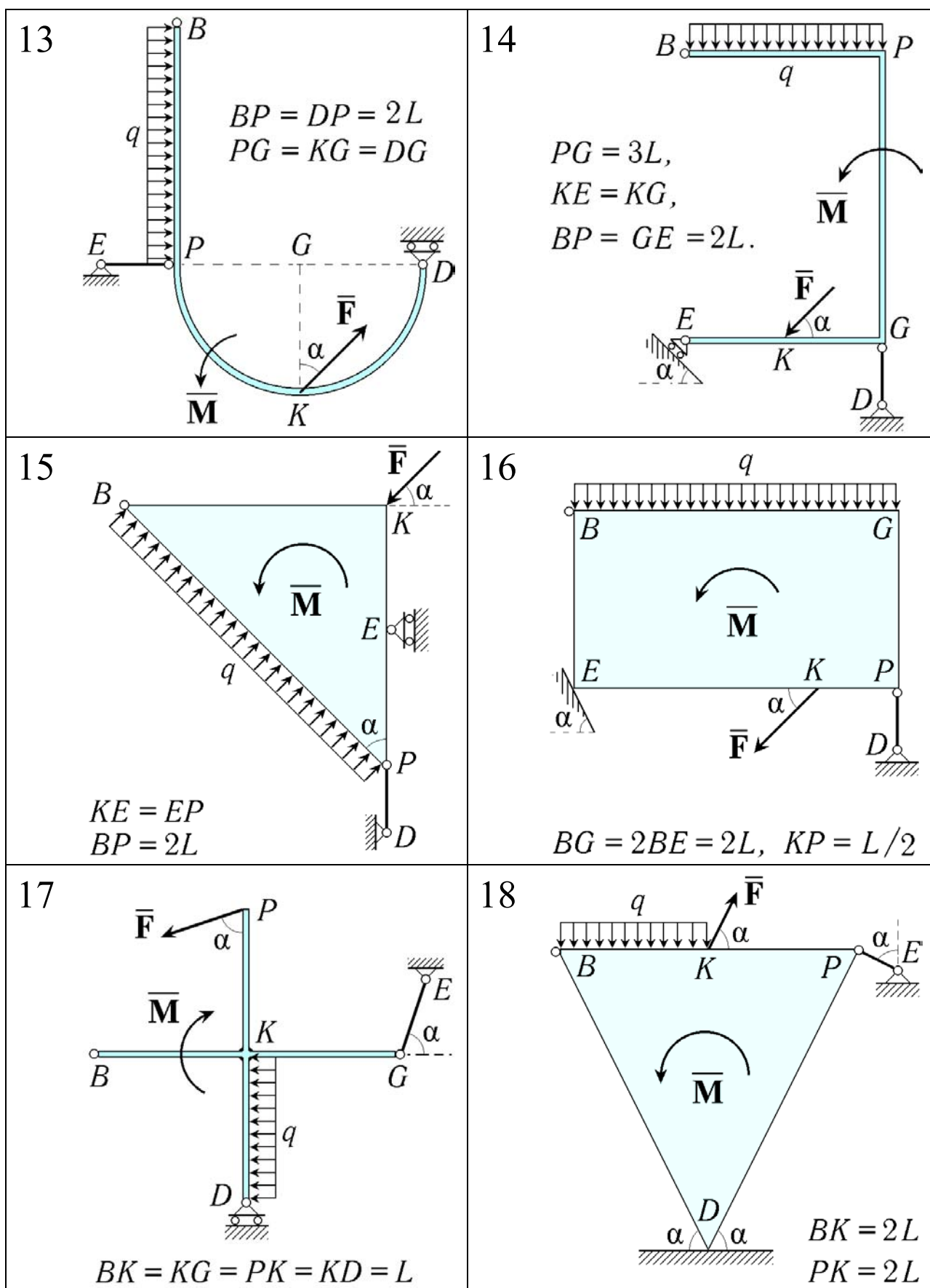
Рис. 14. Группа тел В для ИДЗ (структурные схемы 13 – 18)
