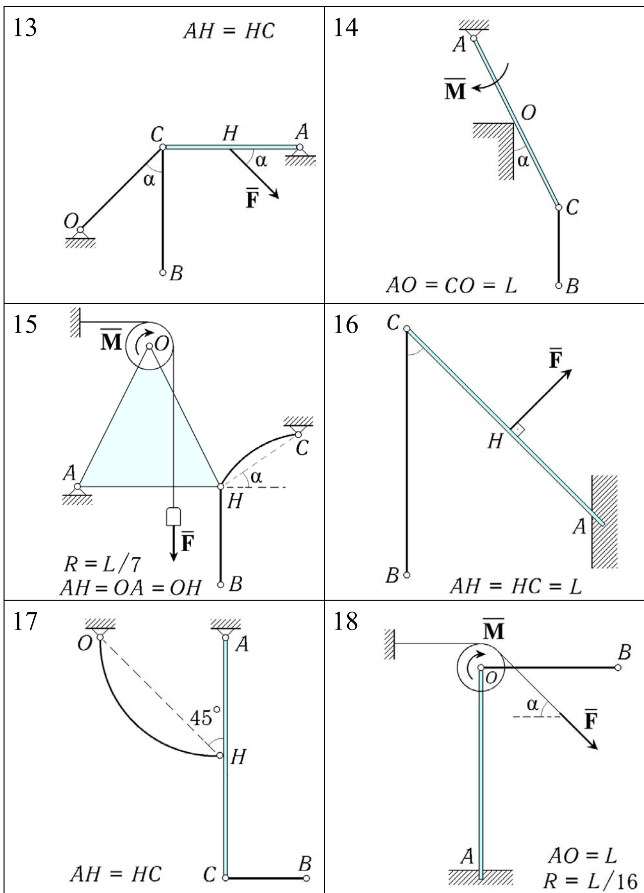
Рис. 10. Группа тел A для ИДЗ (структурные схемы 13 – 18)
