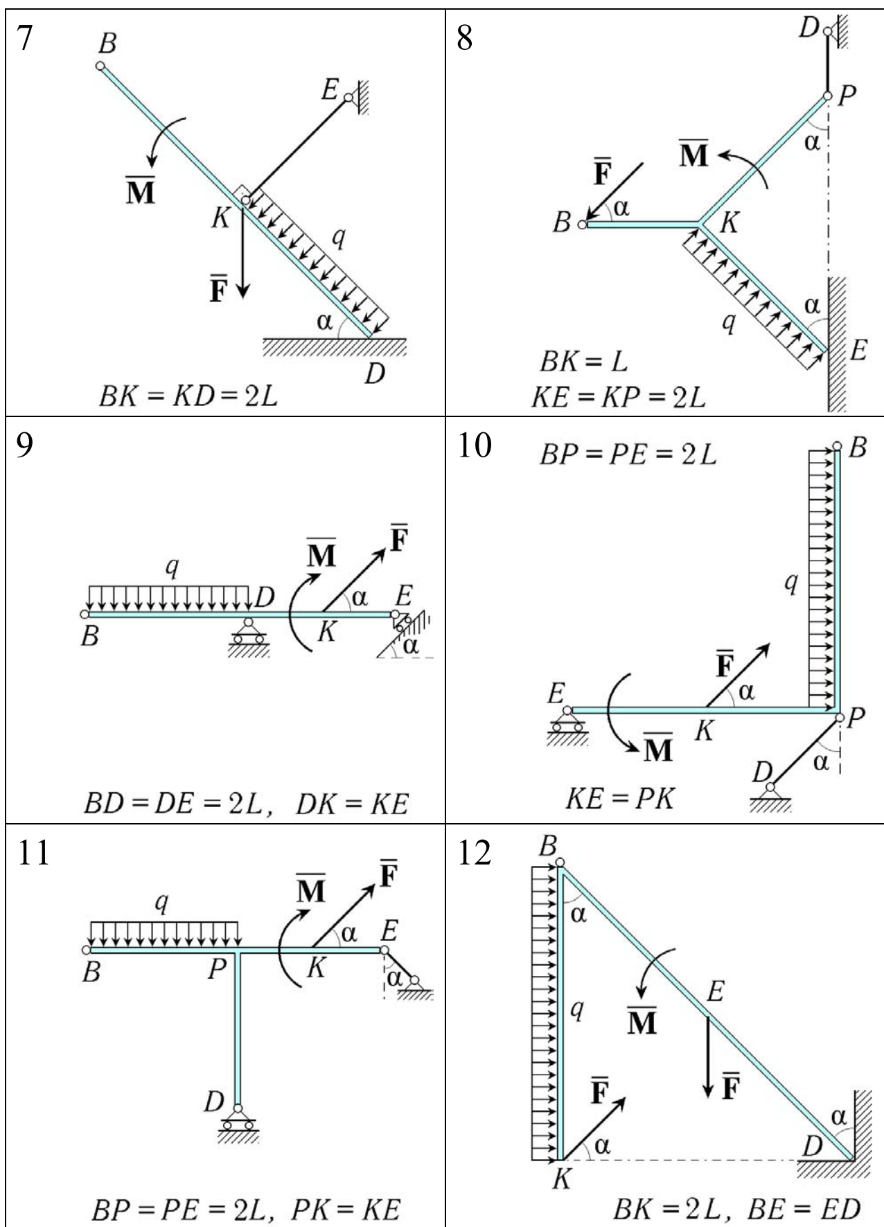
Рис. 13. Группа тел В для ИДЗ (структурные схемы 7 – 12)
