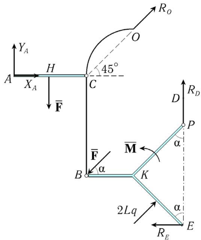
Рис. 17. Система, освобожденная от внешних связей
