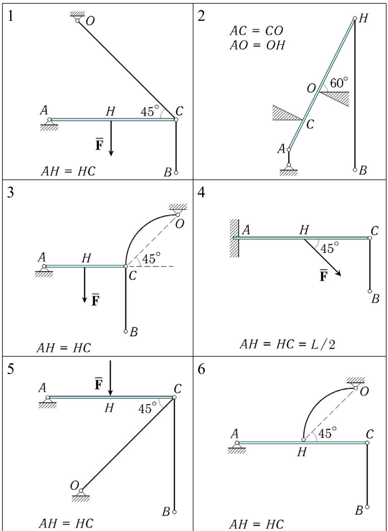
Рис. 8. Группа тел A для ИДЗ (структурные схемы 1–6)
